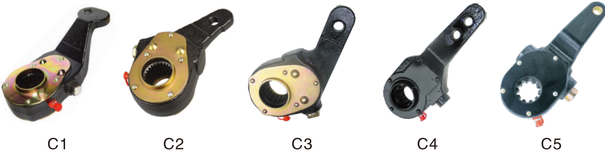
Slack Adjuster
